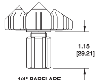
1/4" PARFLARE
