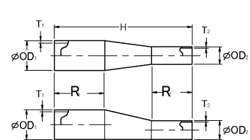
同心/偏心レジュースー [RC] [RE]
