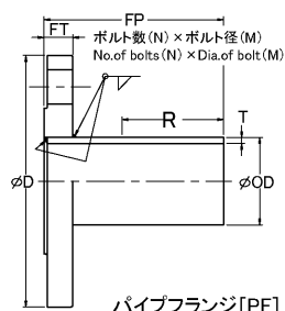
パイプフランジ[PF]
