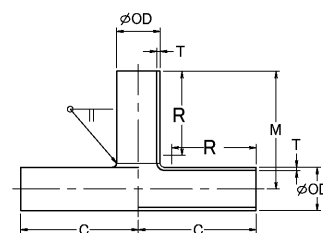
同径ティーズ [E-TEE] [E-TEE-S]
