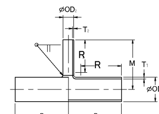
異径ティーズ [R-TEE]
