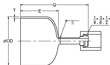
J-キャップ [J-CAP]
