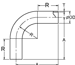
90° ロング/ショートエルボ [90LR] [90SR]
