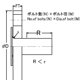
クリーンラップ JIS10K/5K [CLLJ10K][CLLJ5K]
