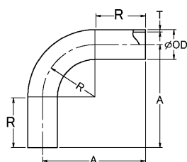
90° ロングエルボ [90LR]
