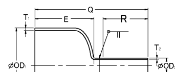
キャップレジュサー [CAP-RC]
