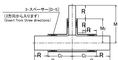
異径ティーズ[D-RT]
