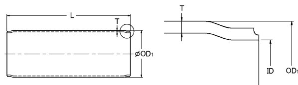
オーバーチューブ(タイプⅡ) [D-OT]
